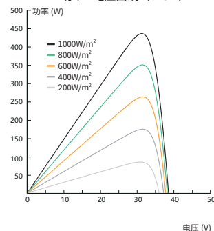
功率 - 电压曲线 (440W)
